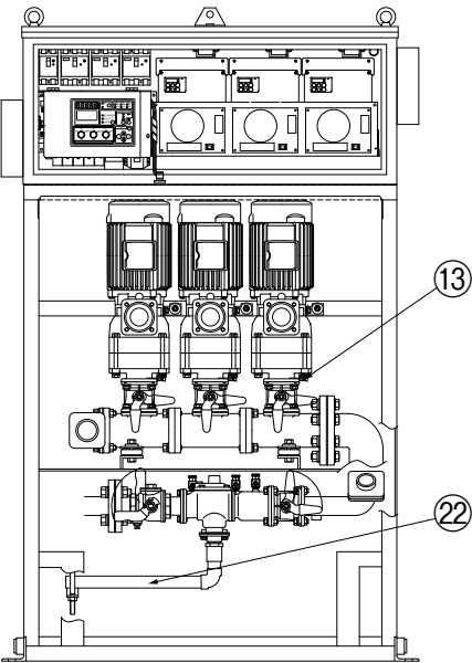
断面BB
