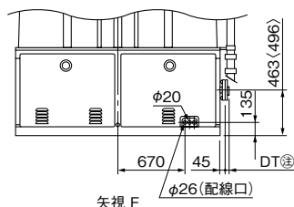
矢視 F
