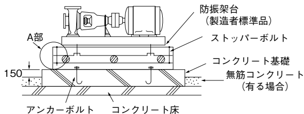
防振基礎
